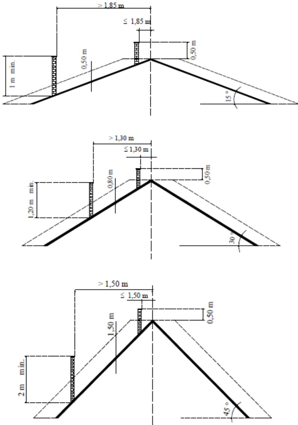
Şekil 31 Çatı uygulamaları
