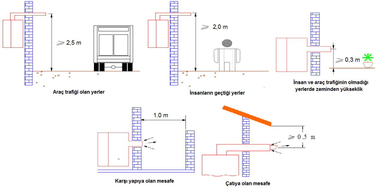
Şekil 19 C tipi cihazların atık ağızlarının yerleşimi
